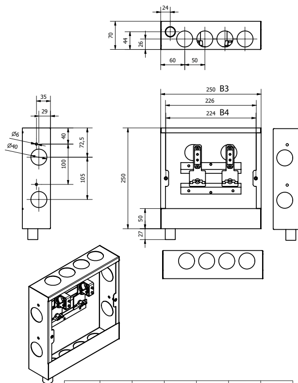
LK Kopplingskåp UNI 250x250
